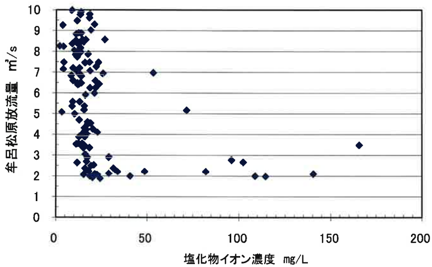
(b) 塩化物イオン濃度－牟呂松原放流量10m 3 /s以下
