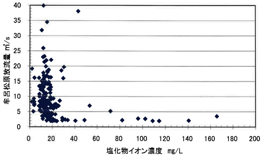
(a) 塩化物イオン濃度－牟呂松原放流量40m 3 /s以下
